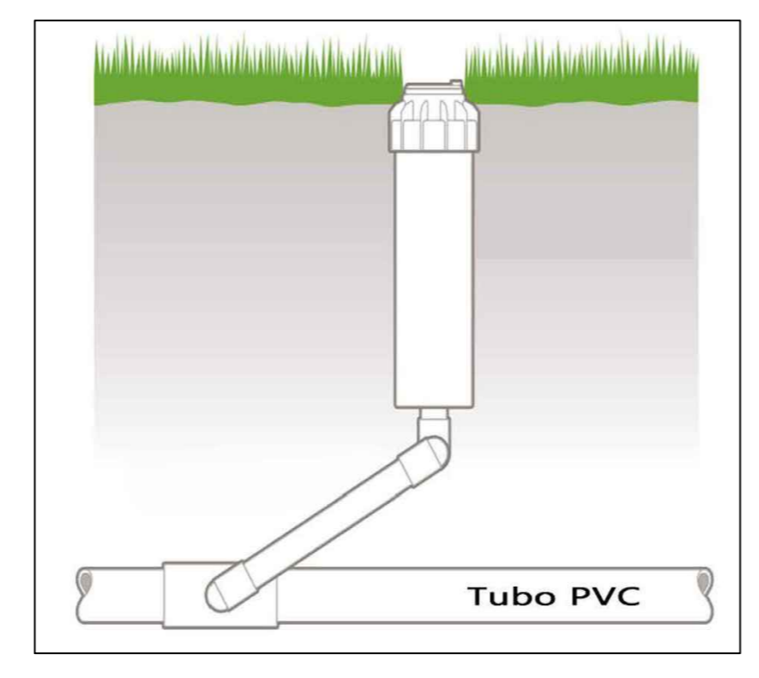
3 DET. ASPERSOR
