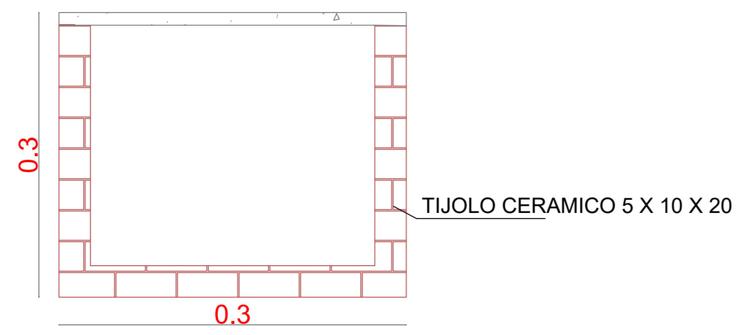
5 Det. Da Caixa de Passagem SEÇÃO 0,30 X 0,30 m
