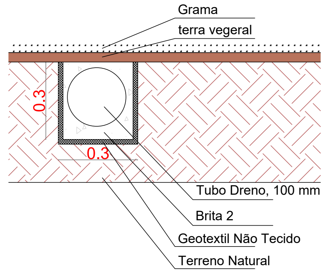
4 DRENO ESPINHA DE PEIXE SEÇÃO 0,30 X 0,30 m
