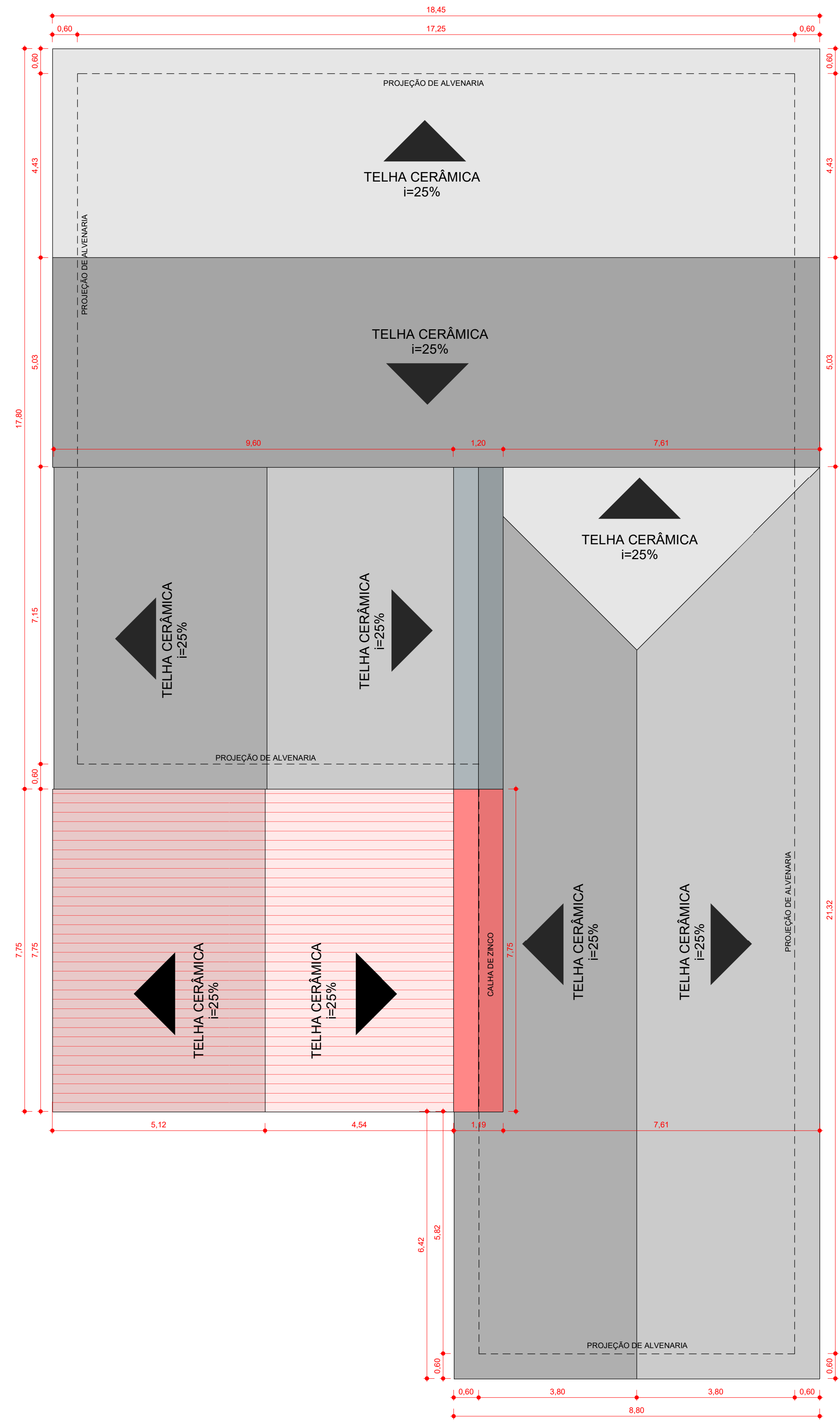
02 Planta de cobertura - Proposta ESCALA - 1 : 75
